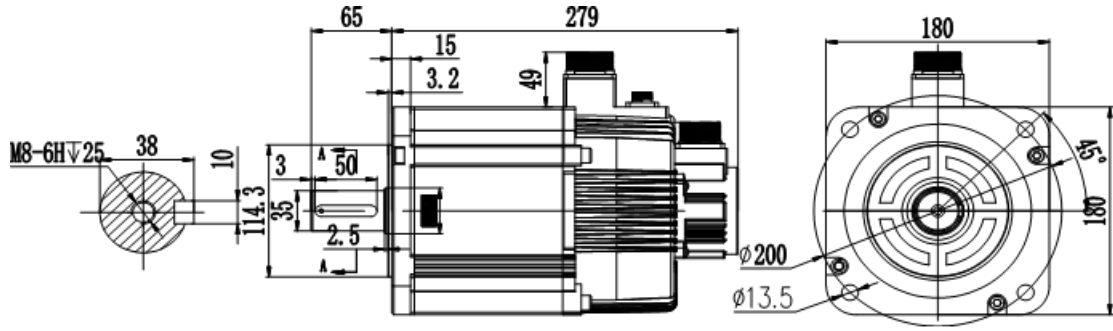
◆ EAM-WH-7515T-U30 7.5kW 带抱闸伺服电机安装尺寸图（单位为 mm）
