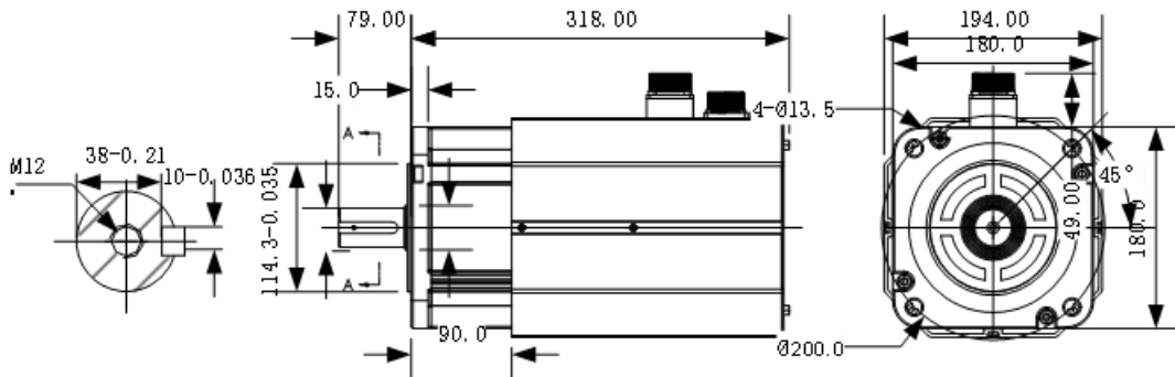
◆ EAM-WH-7515T-U30 7.5kW 带抱闸伺服电机安装尺寸图（单位为 mm）
